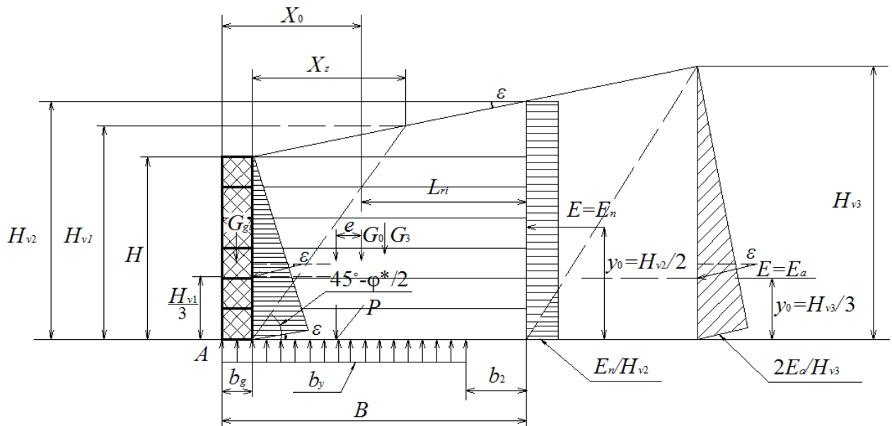
Рисунок И.1 – Розрахункова схема силових впливів на систему «Армогрунтова стіна»
