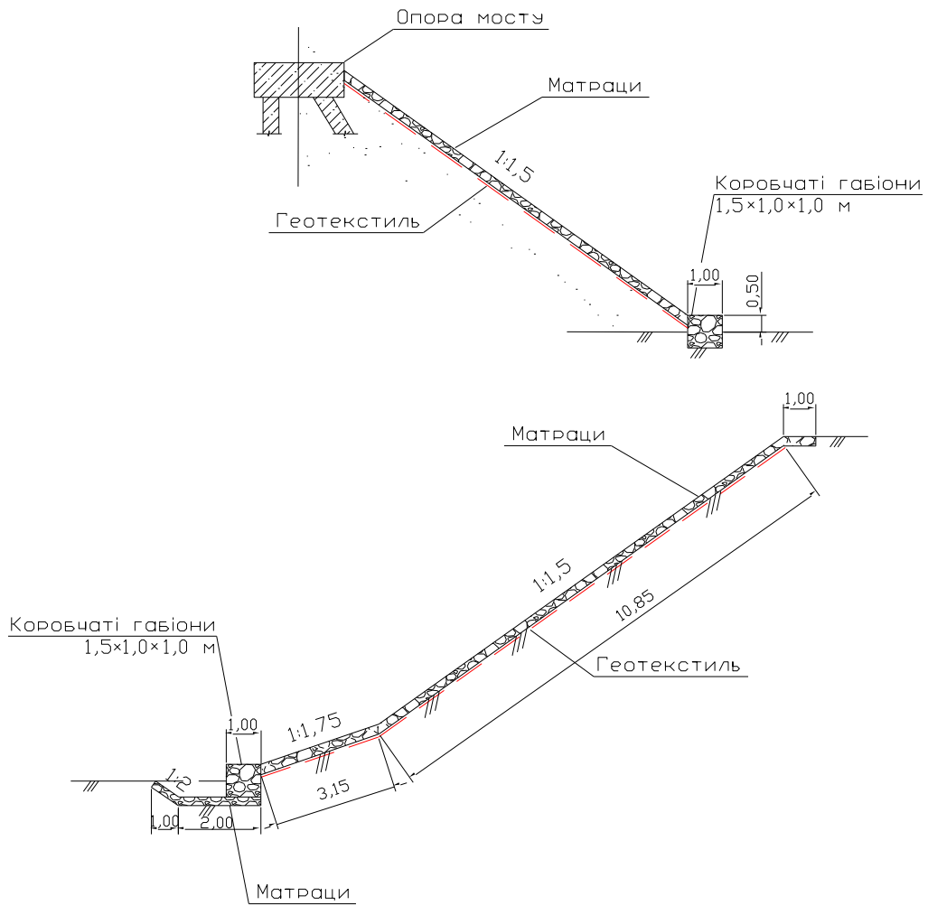
Рисунок Б.6 – Схеми укріплення габійними конструкціями непідтоплюваних укосів: а) підмостових конусів; б) насипів за необхідності влаштування водовідведення
