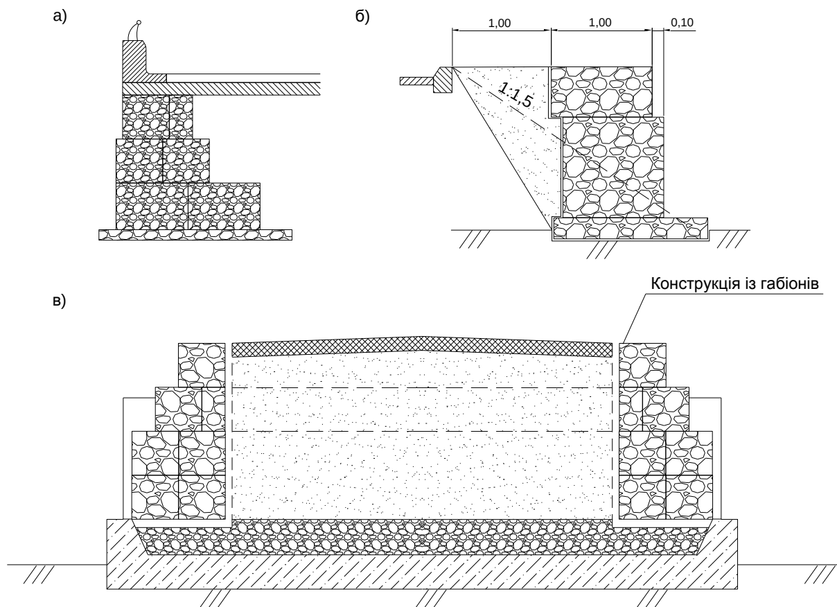
Рисунок Б.3 – Схеми конструктивних рішень заміни укісних частин земляного полотна габіонними підпірно-утримуючими спорудами
