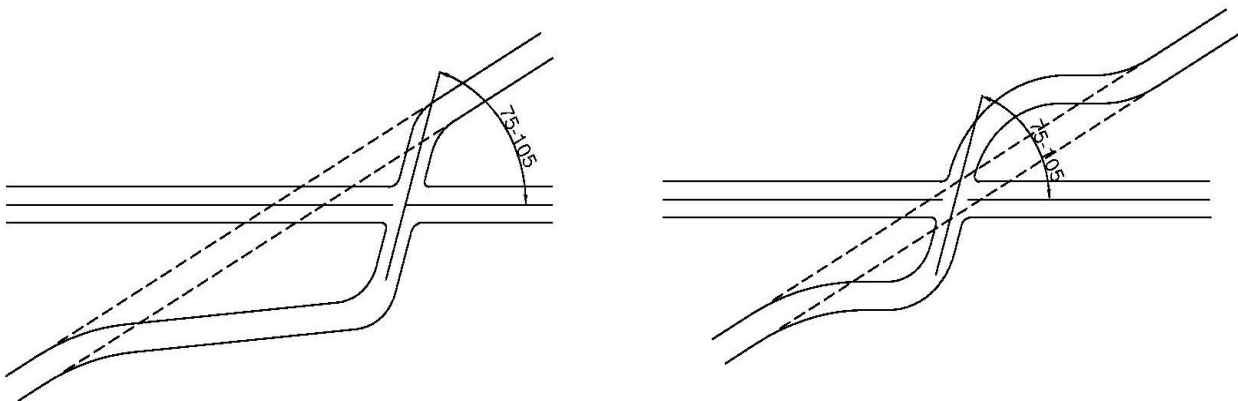
Рисунок 5.1 – Приклади зміни конфігурації розв'язки для зміни кута перехрещення
