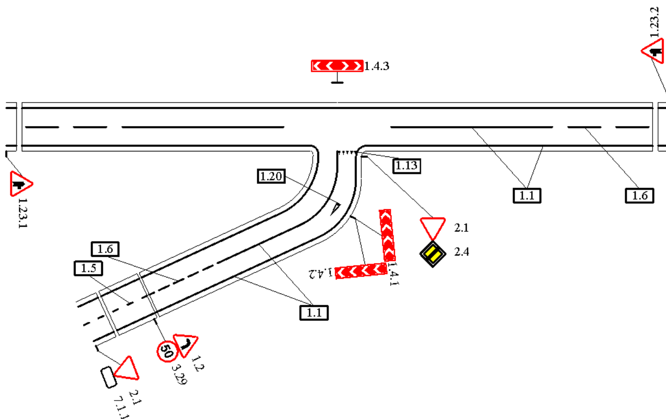
Рисунок Ж.1 – Приклад ОДР при спрямленні кута примикання другорядної дороги
