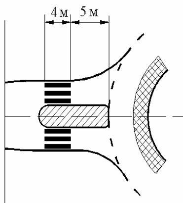
Рисунок 7.2 – Схема розміщення пішохідного переходу з влаштуванням островця безпеки за рахунок прямого островця
