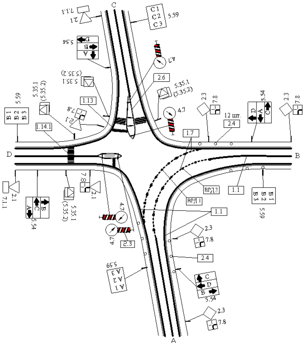
Рисунок Е.1 – Приклад ОДР на транспортних розв'язках, на яких головна дорога змінює напрямку руху
