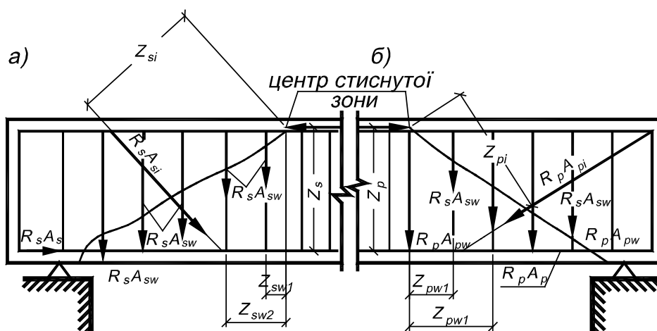
Рис. 3.7 Схема зусиль у перерізі, нахиленому до поздовжньої осі залізобетонного елемента, при розрахунку його міцності на дію згинального моменту а – з ненапружуваною арматурою; б – з напружуваною арматурою
