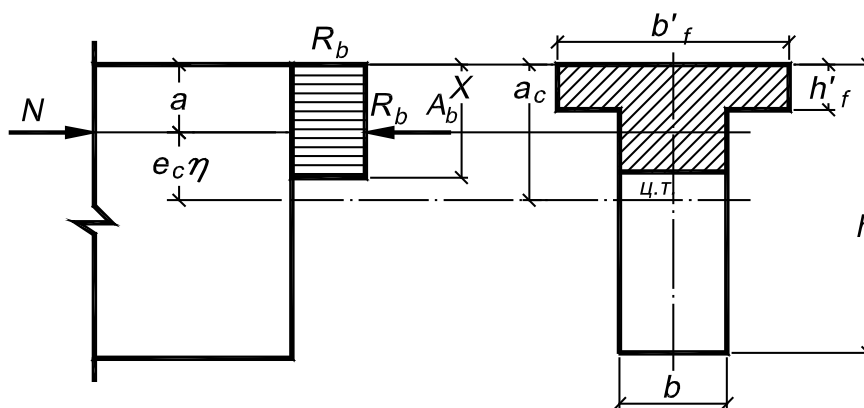
Рис. 3.3 Схема зусиль і епюра напружень у перерізі, нормальному до поздовжньої осі позацинтрово стиснутого бетонного елемента
