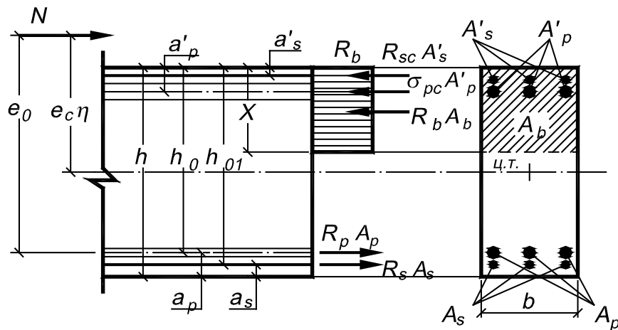
Рис. 3.4 Схема зусиль і епюра напружень у перерізі, нормальному до поздовжньої осі позacentрово стиснутого залізобетонного елемента, при розрахунку його міцності
