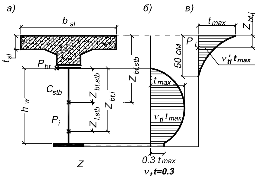
Рисунок 5.1 Поперечний переріз сталезалізобетонної конструкції і розрахункові епюри різниці температур
