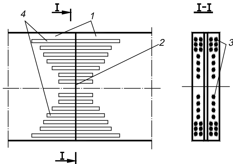
Рис. 6.1 Клеєштирьовий стик
