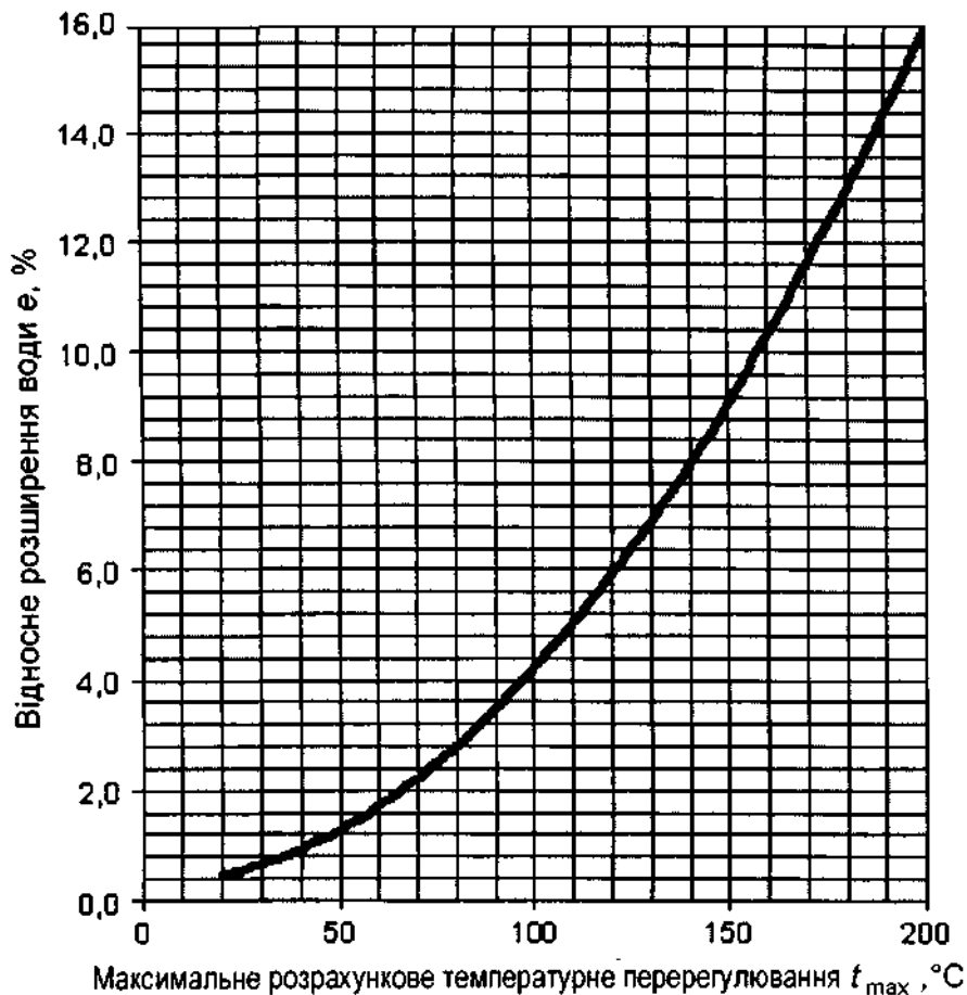
Рисунок Л.2 - Графічна залежність відносного розширення води від максимального розрахункового температурного перерегулювання за температури заповнення 10\text{ }^\circ\text{C}
